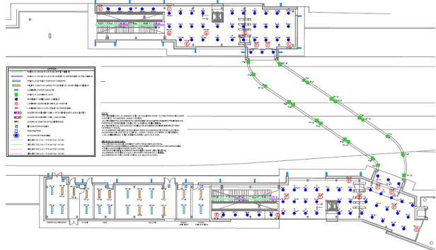
Planta de iluminación de Acceso a andenes
